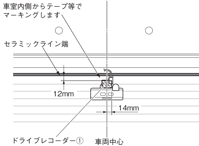
車室内側からバックドアウィンドウを見た図
