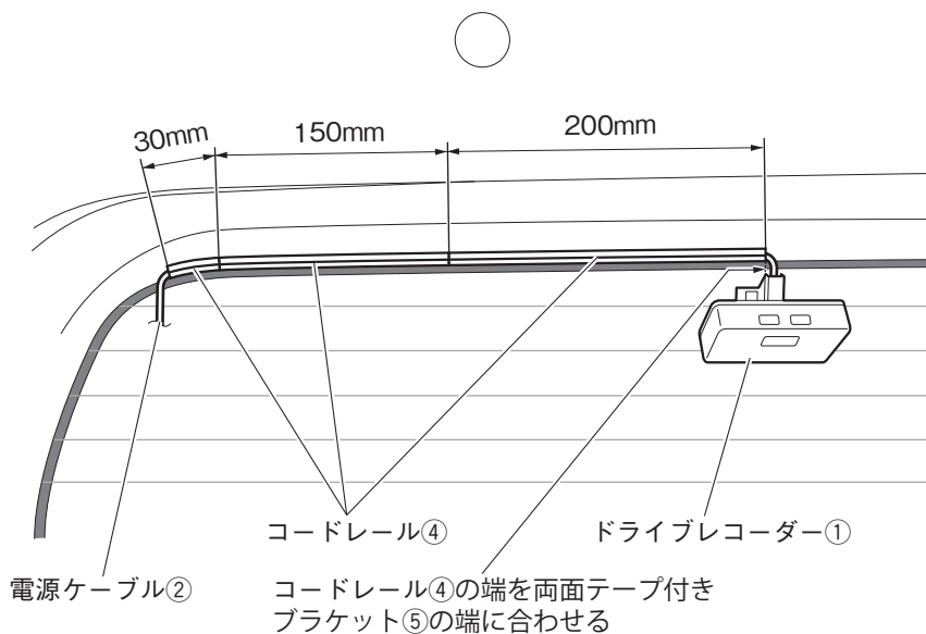
<バックドアガラス上部の配線>
